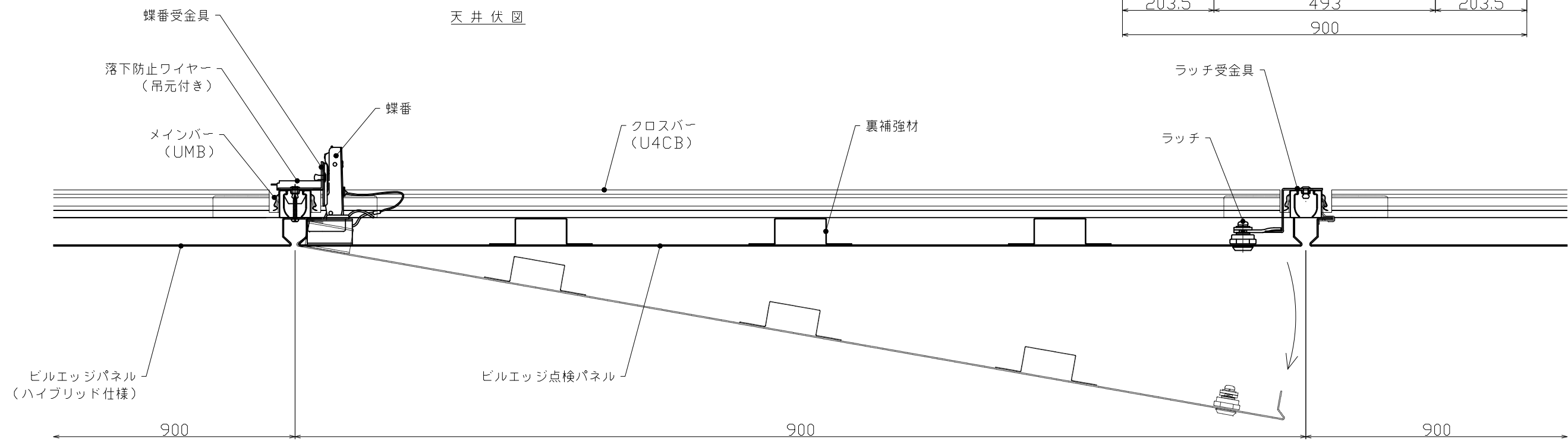
メインバー方向断面図 S=1/4
