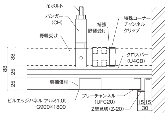
■壁際納まりメインバー方向断面図
