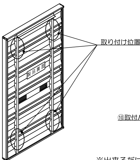
取り付け位置 ※たて格子例
