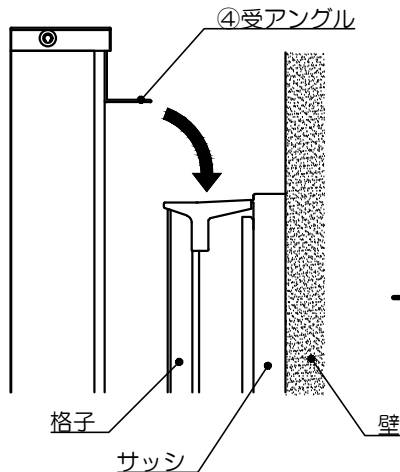
図：乗せ掛けのイメージ
