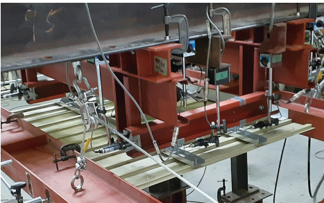
写真1 試験状況(野縁直交方向)
