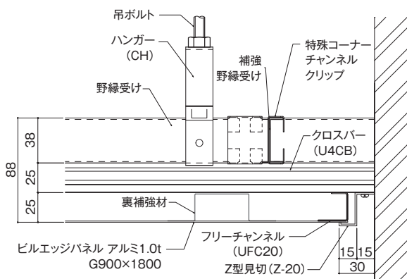
■壁際納まりメインバー方向断面図
