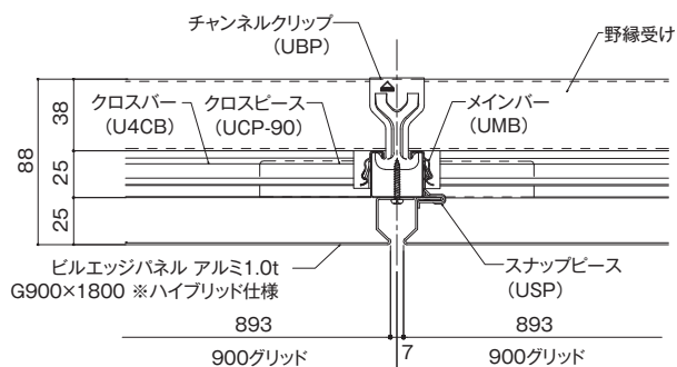
■メインバー方向断面図
