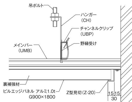
■壁際納まりクロスバー方向断面図
