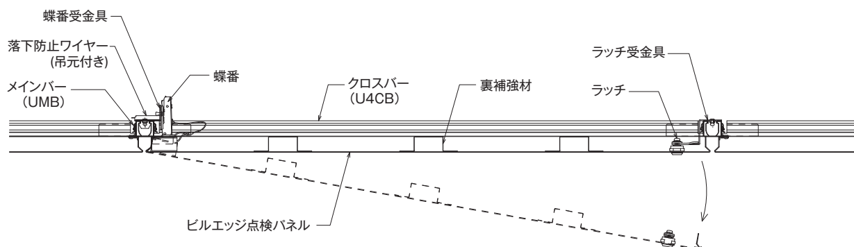
■メインバー方向断面図
