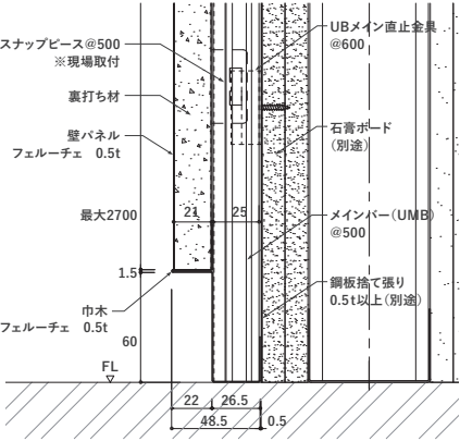
【縦断面図】
