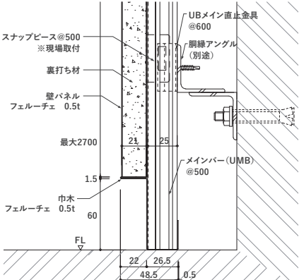
【縦断面図】
