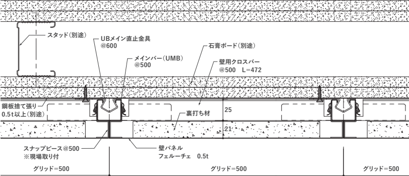
【横断面図】
