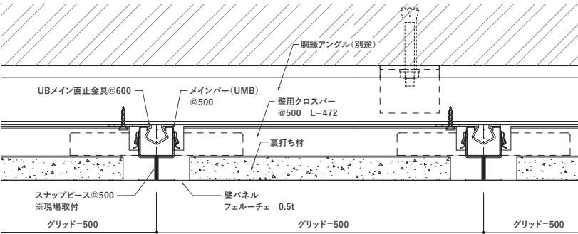
【横断面図】
