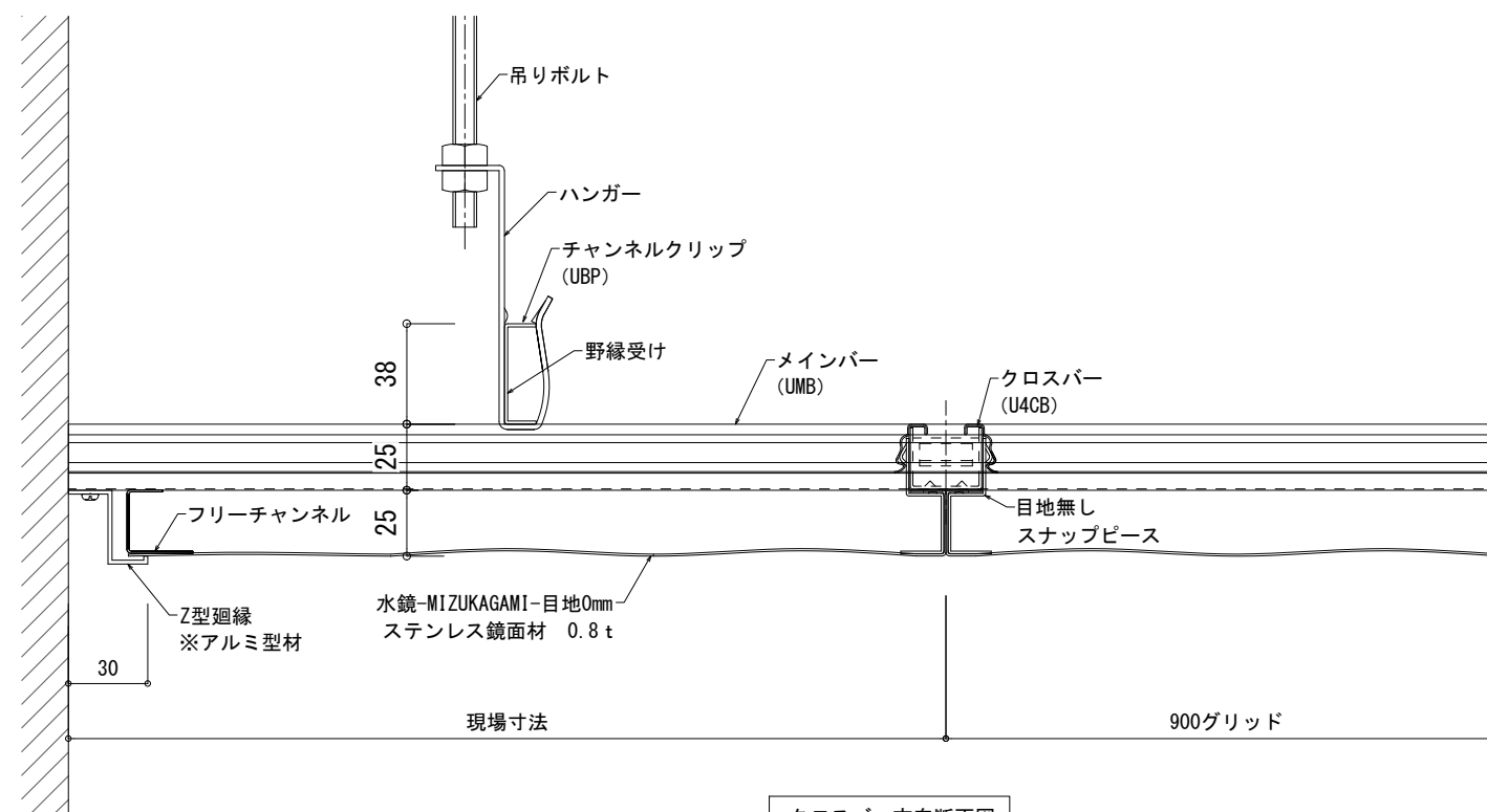
クロスバー方向断面図
