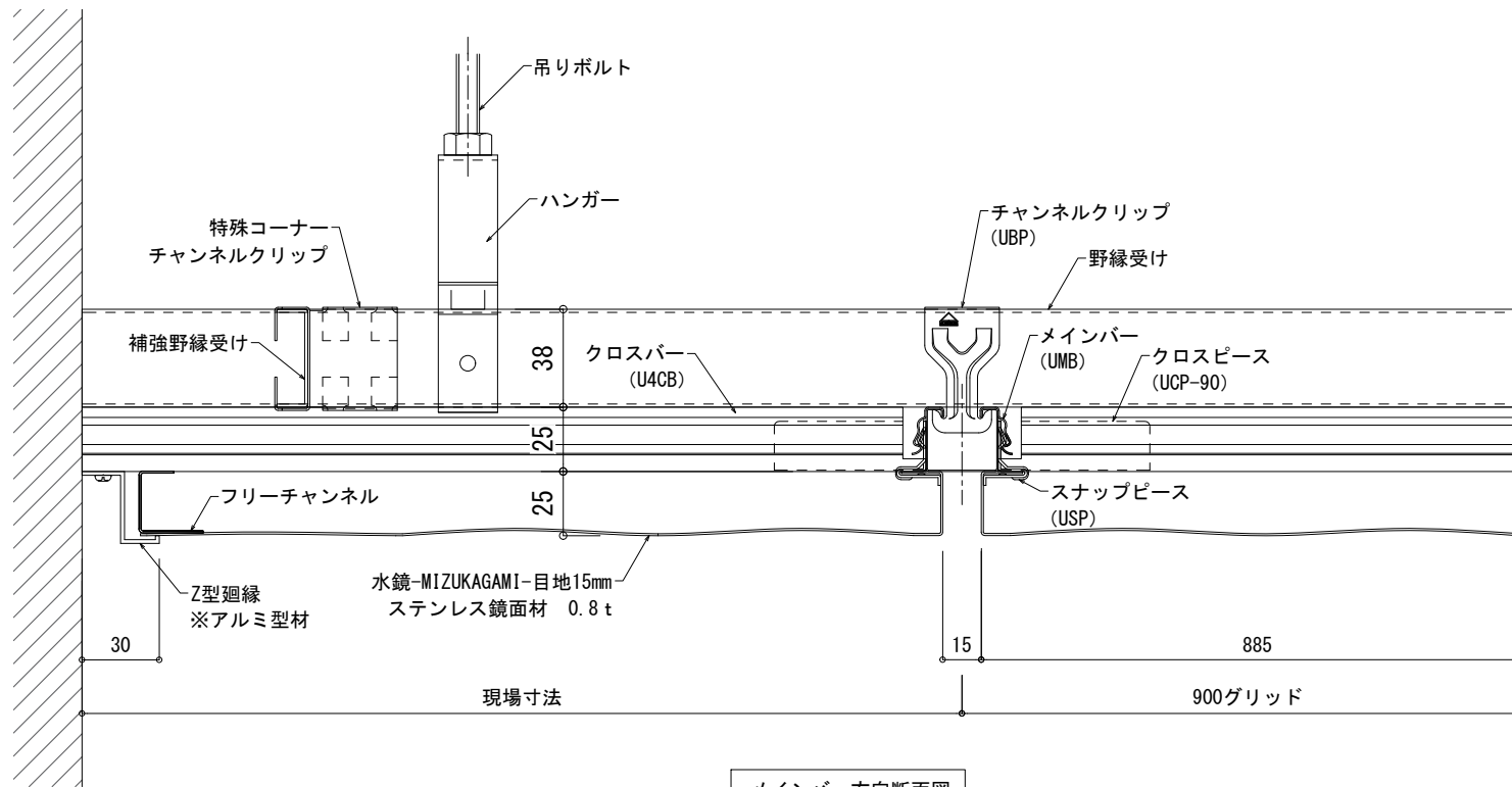
メンバー方向断面図
