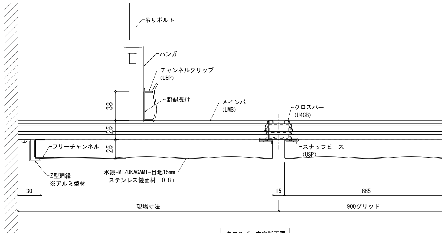
クロスバー方向断面図
