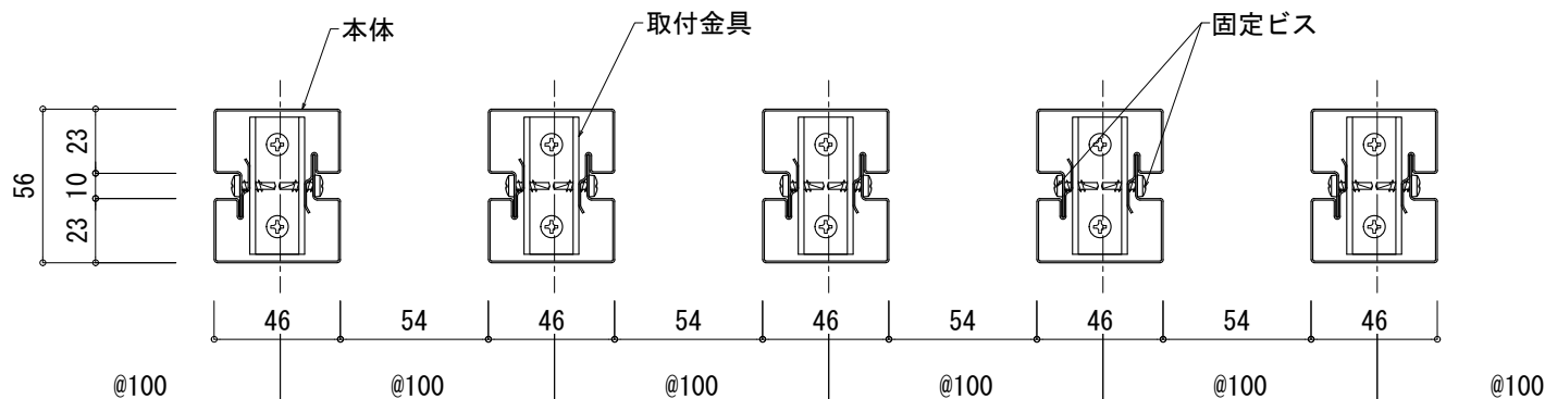
WALLライン-46 基本断面図
