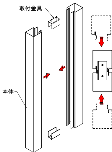
WALLライン-52 基本断面図
