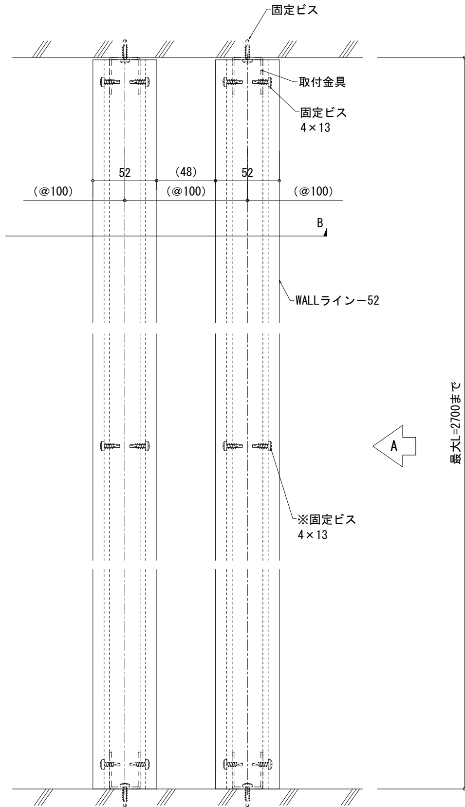
立面図
