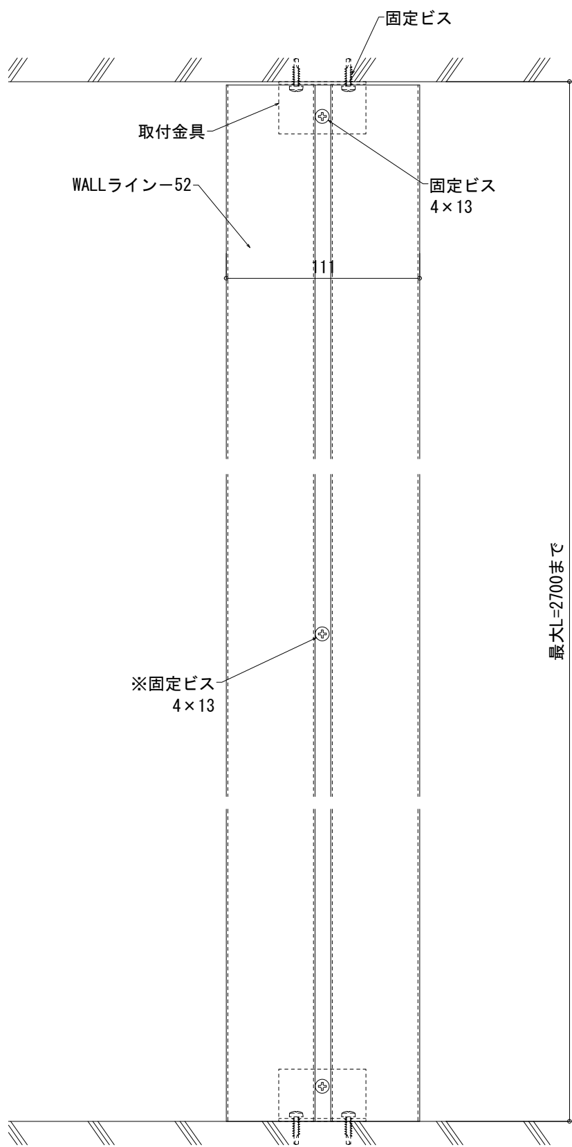
A矢視図
