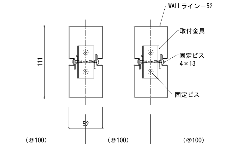
B断面詳細図
