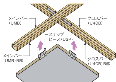
【スナップイン工法図】
